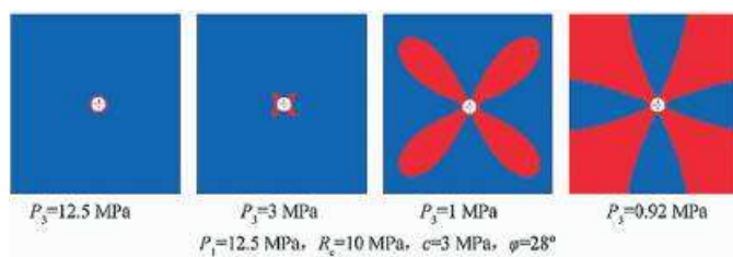
Рис. 2 Зоны развития пластических деформаций (красный цвет) вокруг выработки при изменении соотношения напряжений в массиве P_3/P_1
